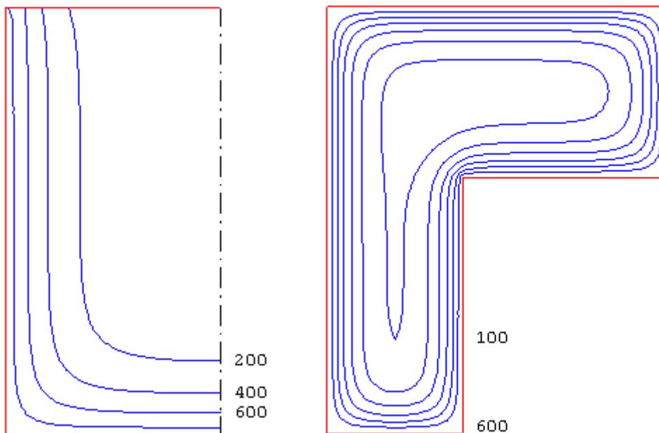
Рис.9. Изотермы
