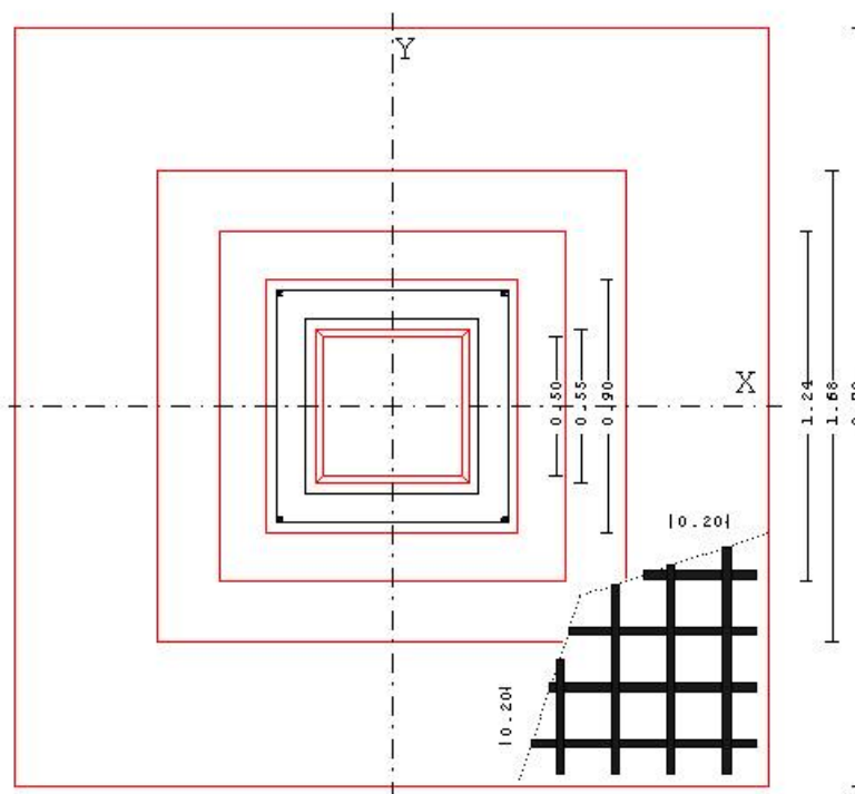
Схема фундамента вид сверху И = 1 : 23
