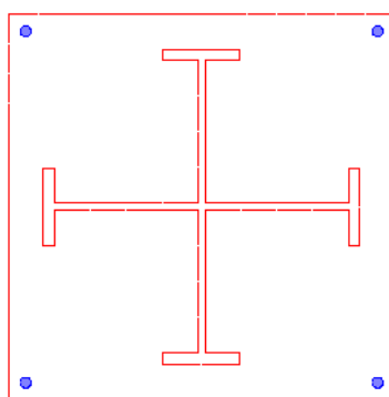
Рис. 9. Трубобетонные сечения
