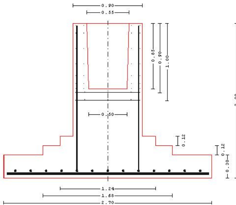
Схема фундамента вид сбоку И = 1 : 23
