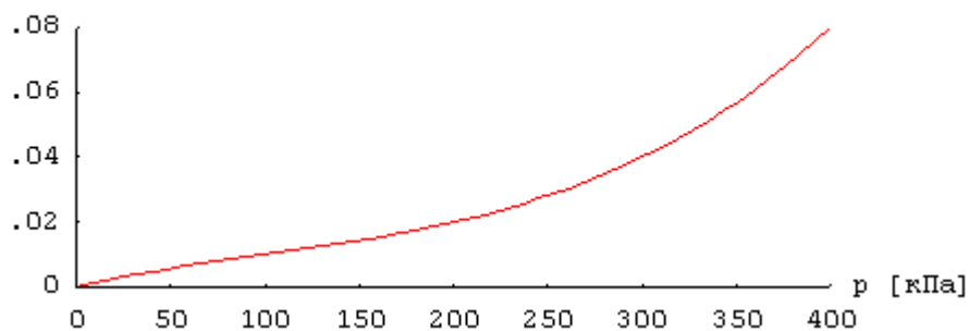
График зависимости \varepsilon_{st} = f(p)
