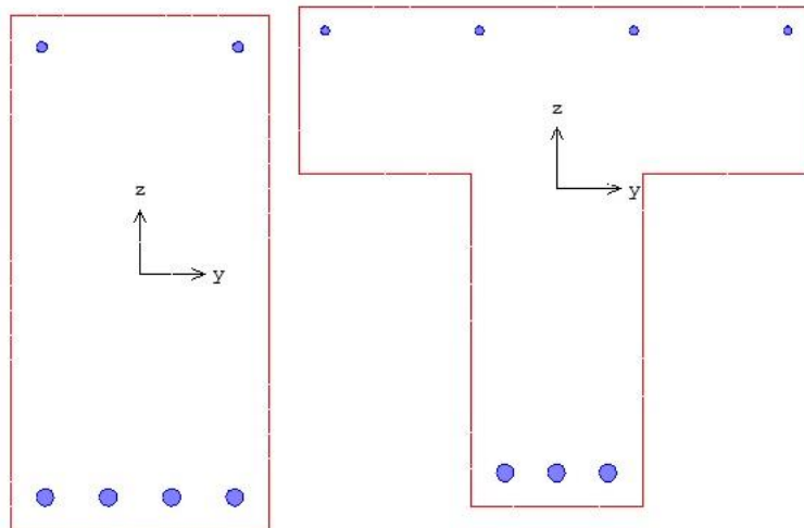
Рис.1 Сечения балки
