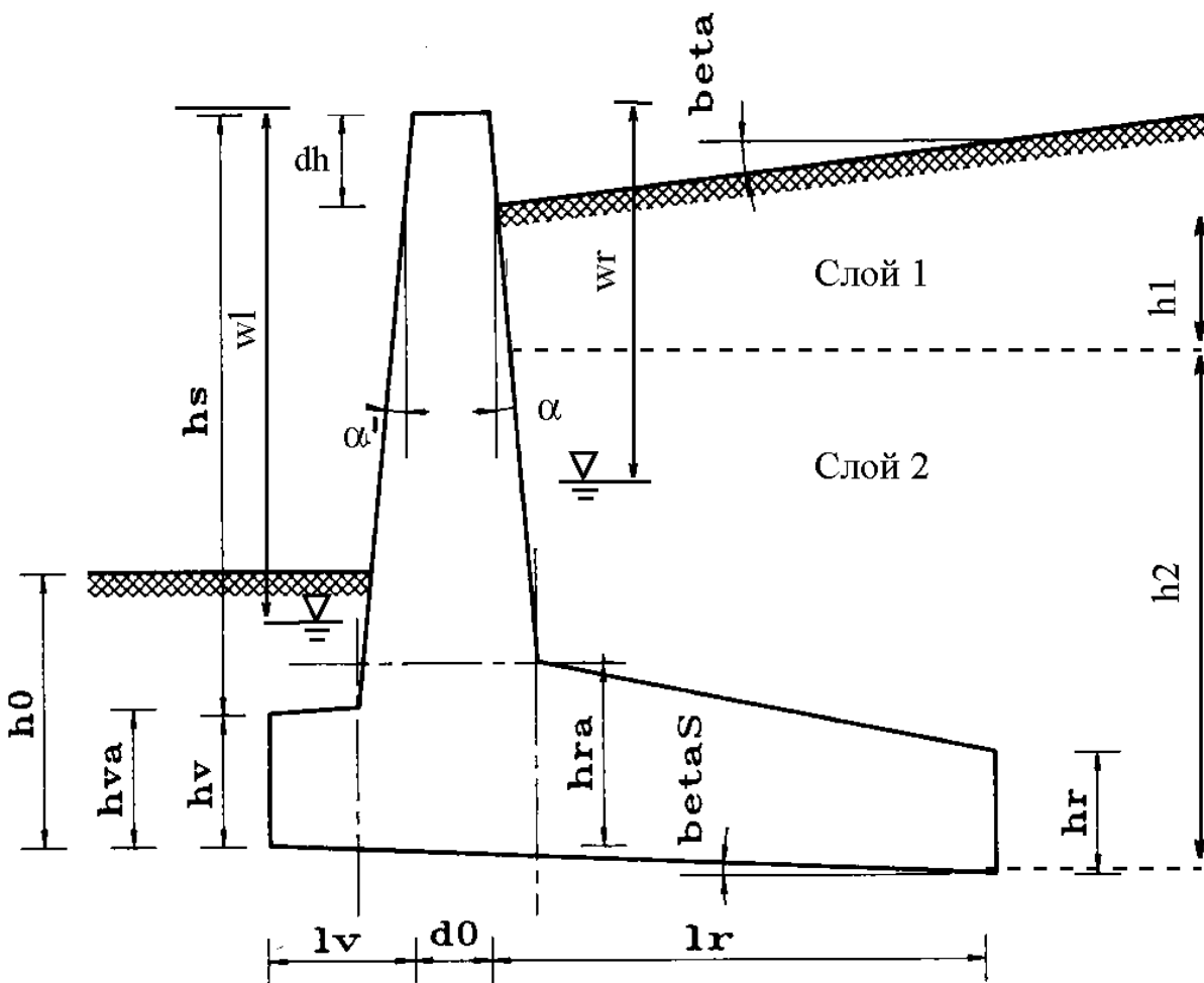
Рисунок 1: Расчетная схема
