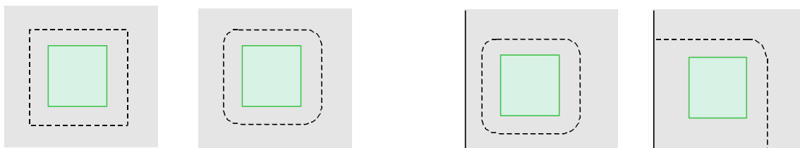
а) варианты построения большего основания пирамиды продавливания
