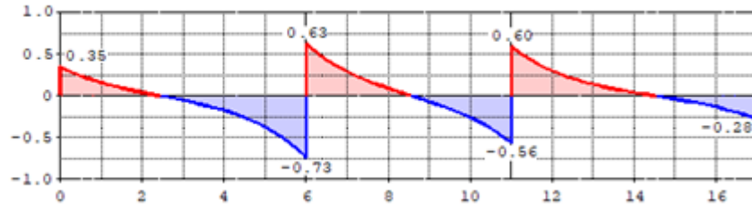
Крутящий момент M_x , [кНм]
