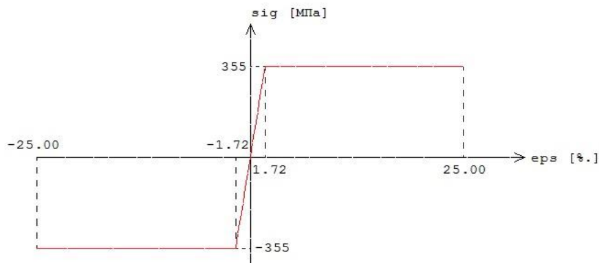
Рис.5. Диаграмма деформирования стали С375 при нормальной температуре
